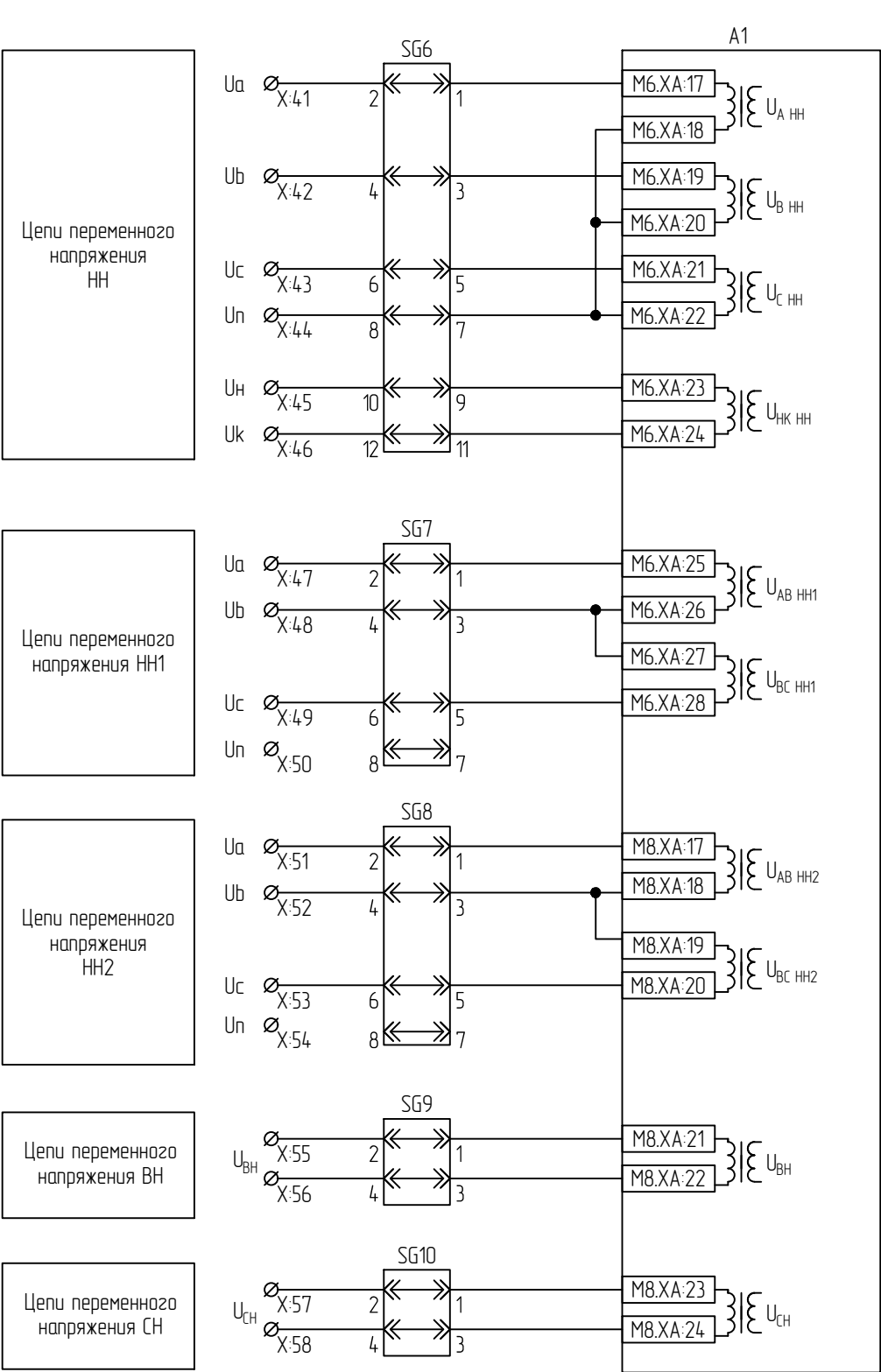
Цепи переменного и напряжения А1
