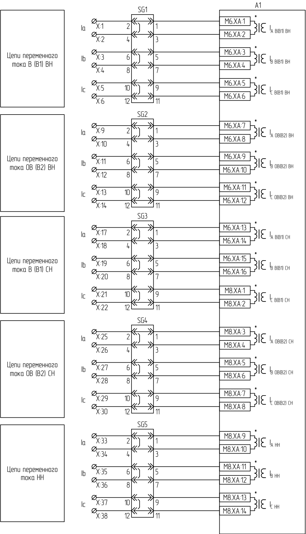
Цепи переменного тока А1
